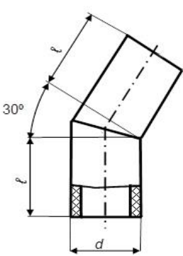
відвід 30° одностиковой
