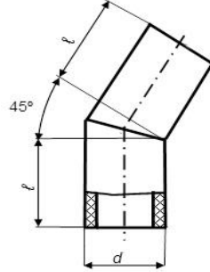
відвід 45° одностиковой
