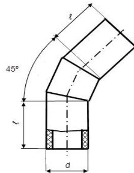
відвід 45° односекційний
