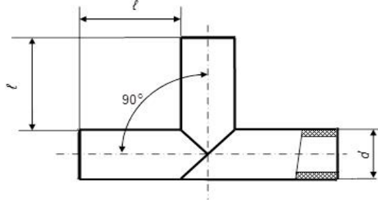
Трійник
