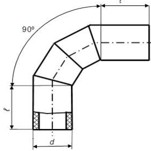
відвід 90° двосекційний
