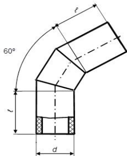
відвід 60° односекційний
